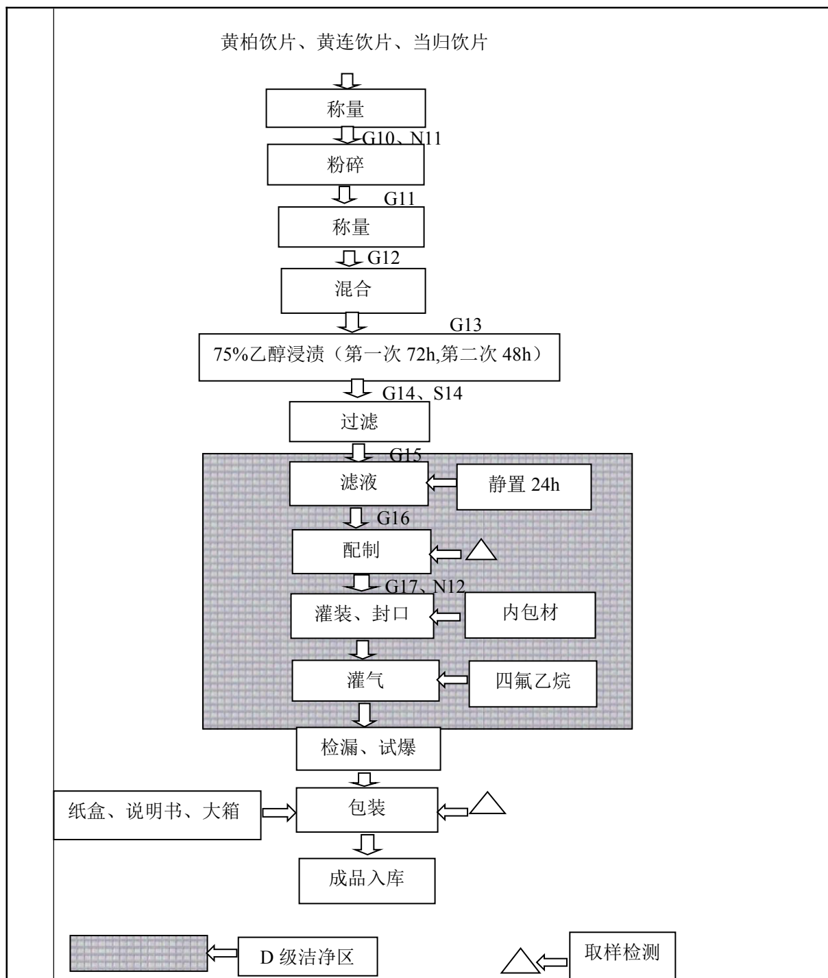
图 2-7 湿疡气雾剂生产工艺流程及排污节点图
